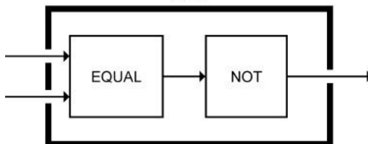
XOR:
