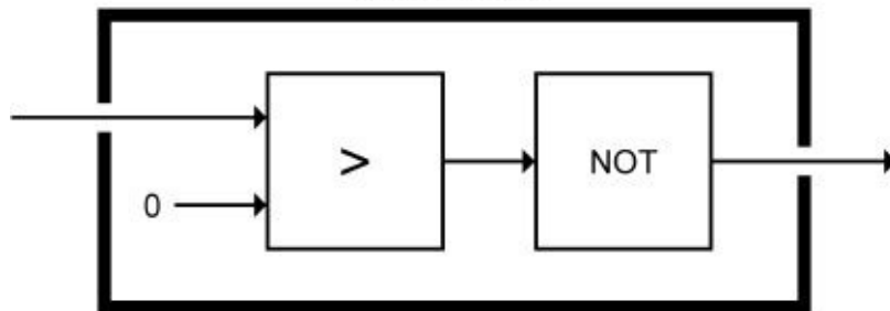
NOT-PLUSP:
