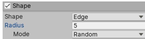
Figure 7.22 – Edge shape
